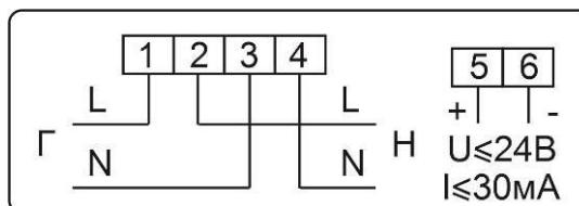
Рисунок Б.10 – Схема включения счетчиков в корпусах W1 с одним дискретным выходом
