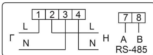
Рисунок Б.26 – Схема включения счетчиков в корпусах W6, W6b, W9 с интерфейсом RS-485
