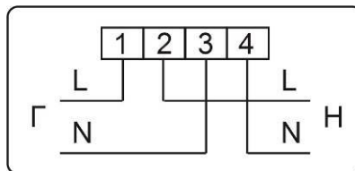
Рисунок Б.9 – Схема включения счетчиков в корпусах W1
