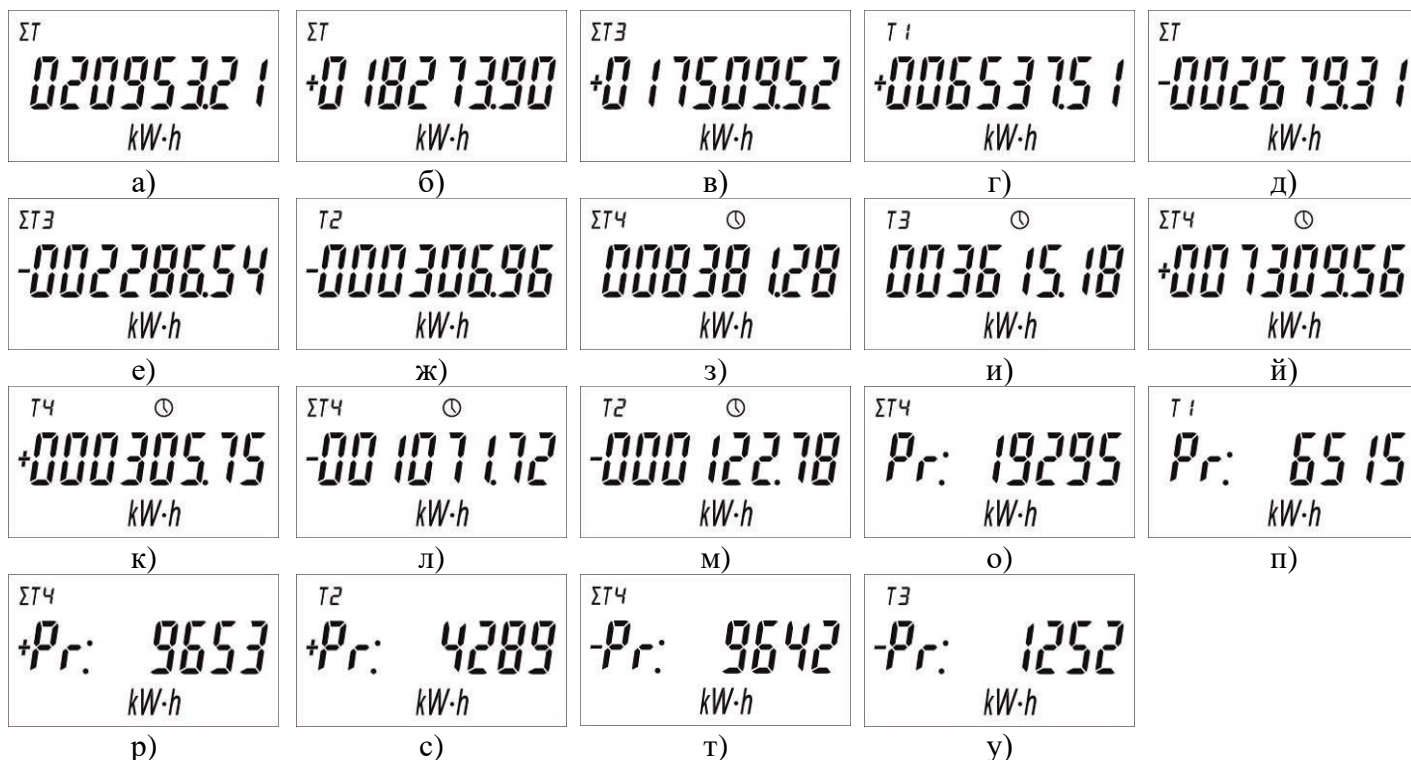
Рисунок 3.5 – Программируемые режимы индикации счетчика
