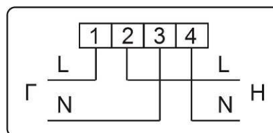
Рисунок Б.15 – Схема включения счетчиков в корпусах W2
